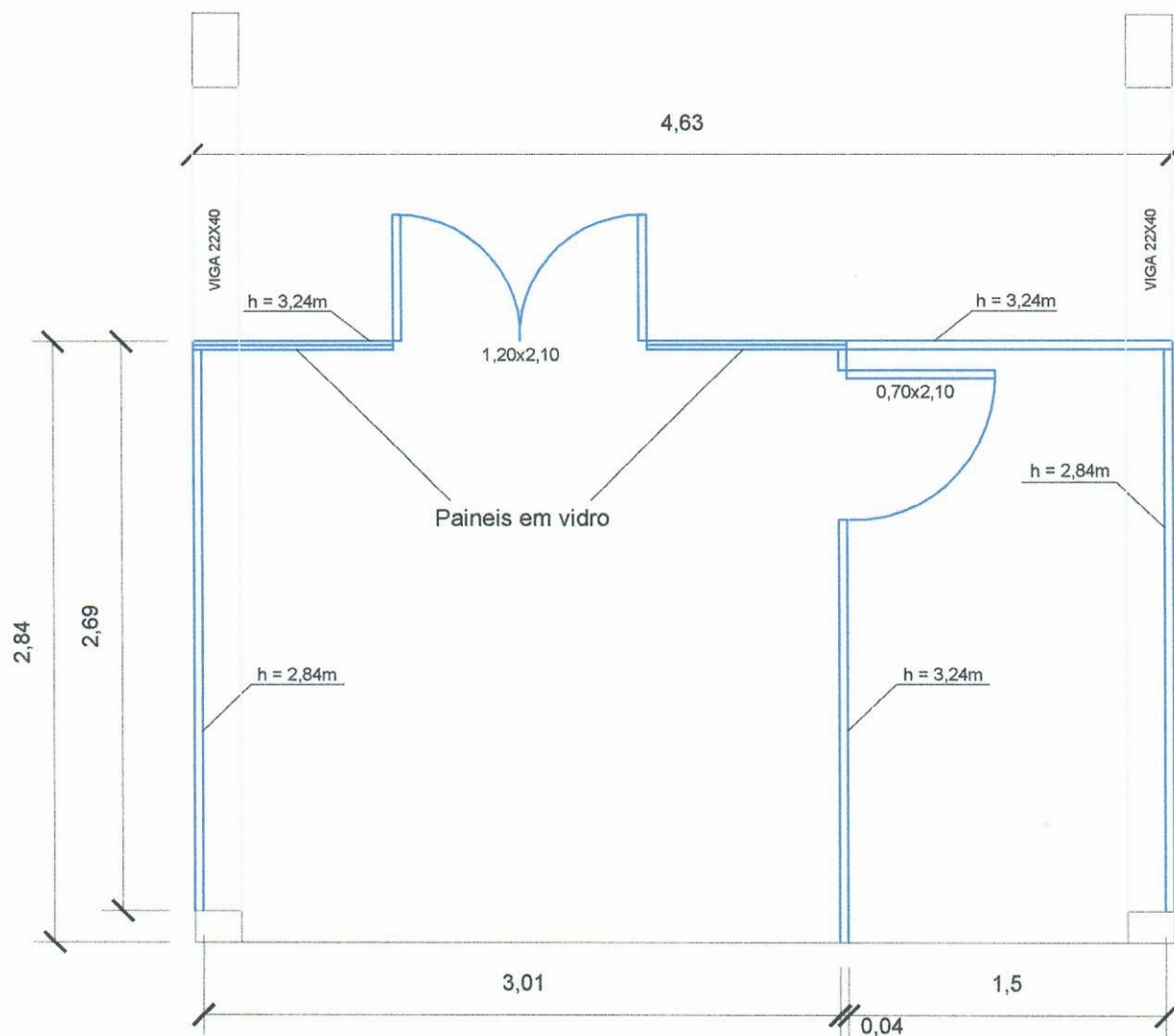
Planta Baixa
